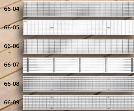
66-10 ACO Profiline Holzterrassenrinne: Maschenroste in versch. Ausführungen
