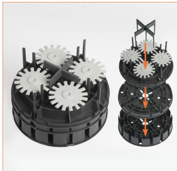
MultiLager, MultiLager+Plus und VarioLager mit Fugenkreuz zur Rückdrehsicherung
