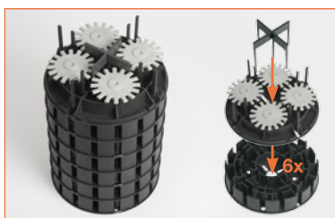
Maximale Höhe: VarioLager mit Rückdrehsicherung und 6x MultiLager+PLUS
