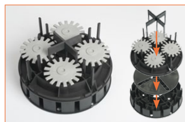
VarioLager mit Rückdrehsicherung, Maxi-Ausgleichsscheibe und MultiLager+PLUS
