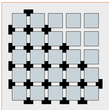
Kreuzverband
