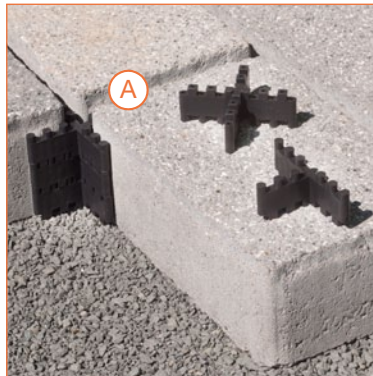
Fugen-T-Stücke verlegen
