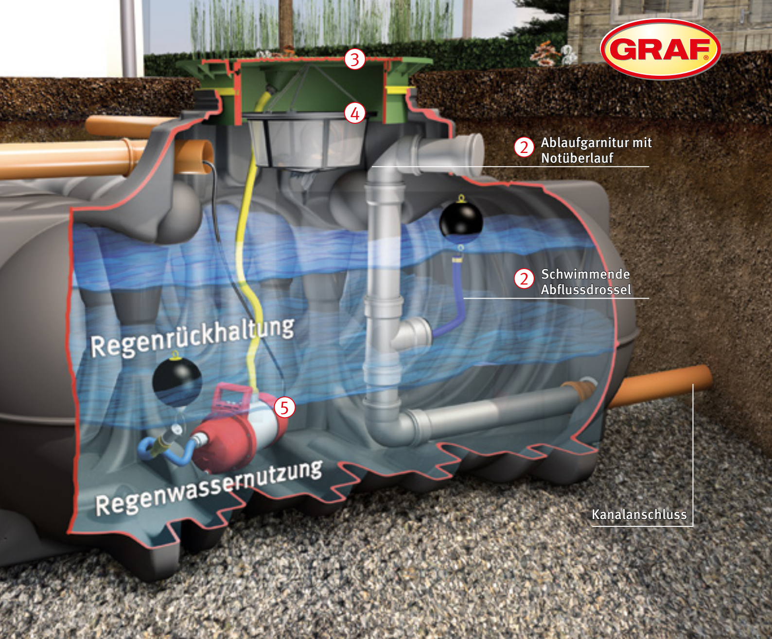
Abbildung zeigt Platin Retentionszisterne Plus für die Gartenbewässerung
